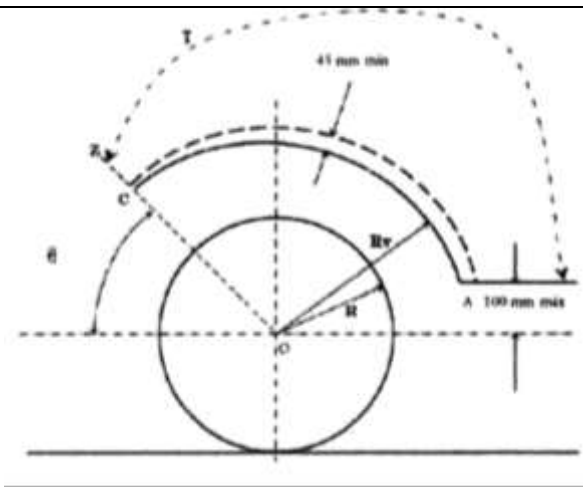
Figura N°4. Dimensiones y cobertura del guardafangos.
